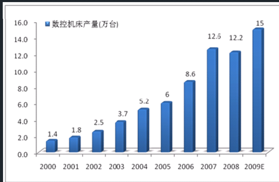
图：2000-2009年中国数控机床年度产量变化
