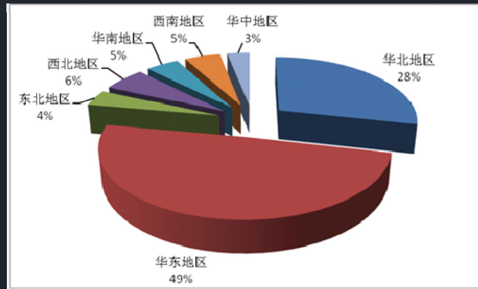
图：2009年中国数控机床分区域产量分布
