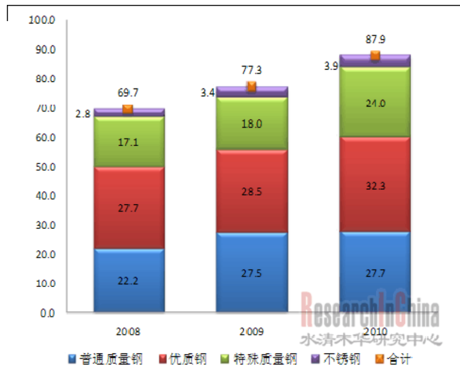
图：2008-2010年中国32家特钢企业产量情况（单位：百万吨）
