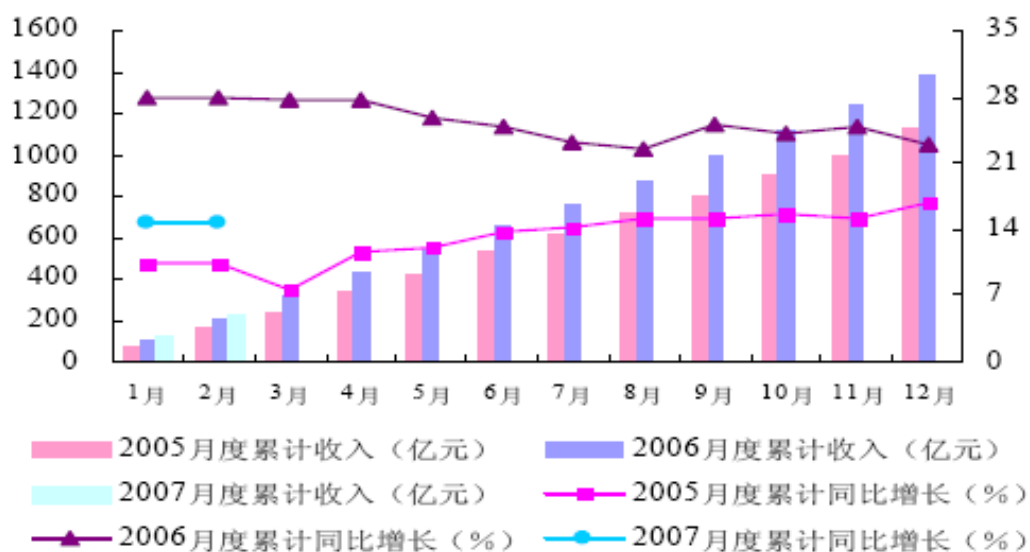
化学制剂行业月度累计销售收入及同比增长情况
